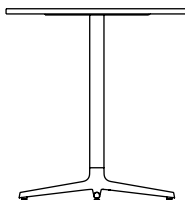
Allez table 4L H75 Ø70 cm H: 75 x Ø70 cm
